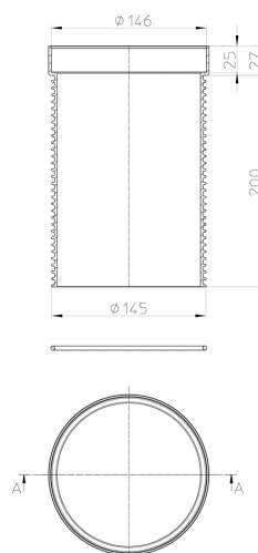
Schnitt A-A
